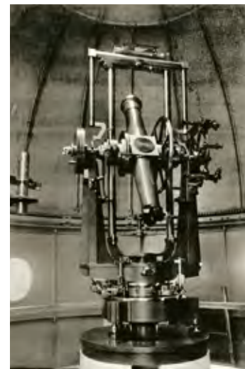
L'altazimut de Gautier dans sa coupole. Photographie Auguste Lebeuf, 1892.
